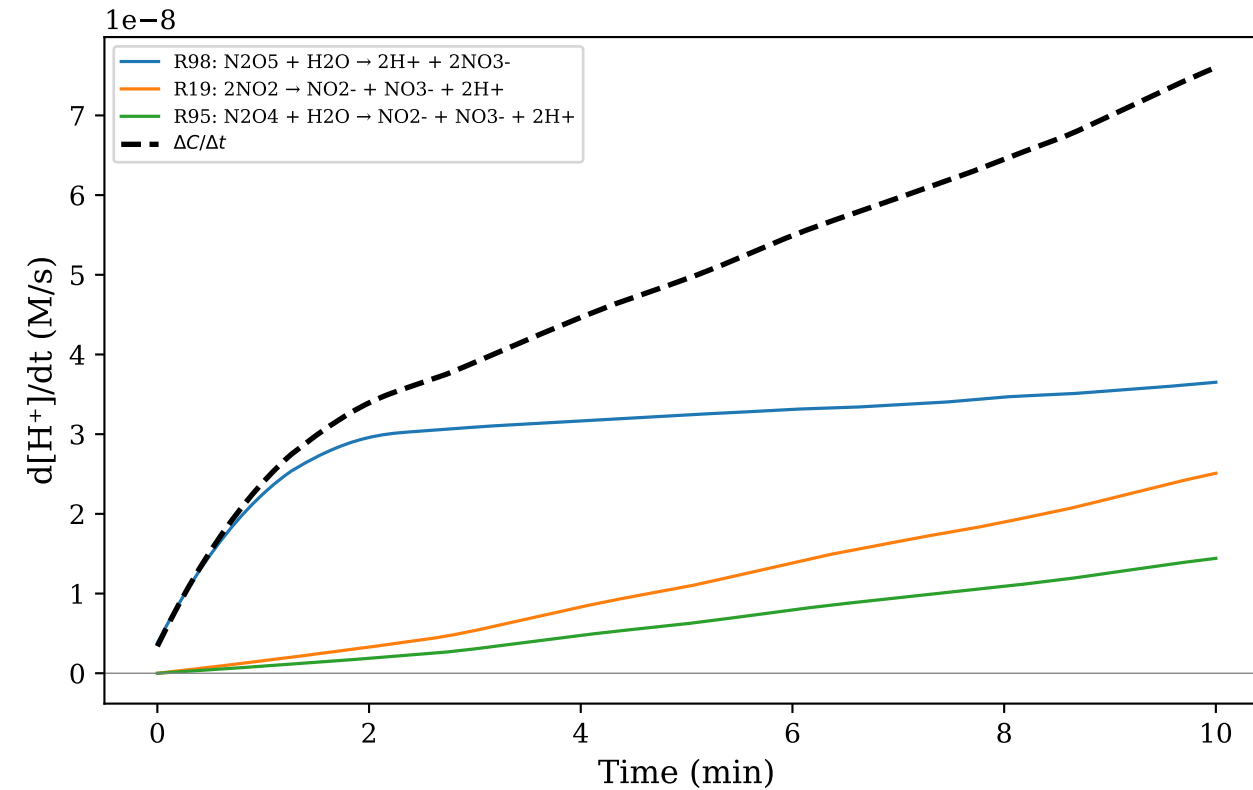
(d) H + [final=28.99 μM]
