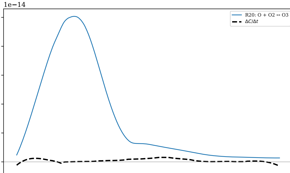
(a) O [final=-0.01 pM]
